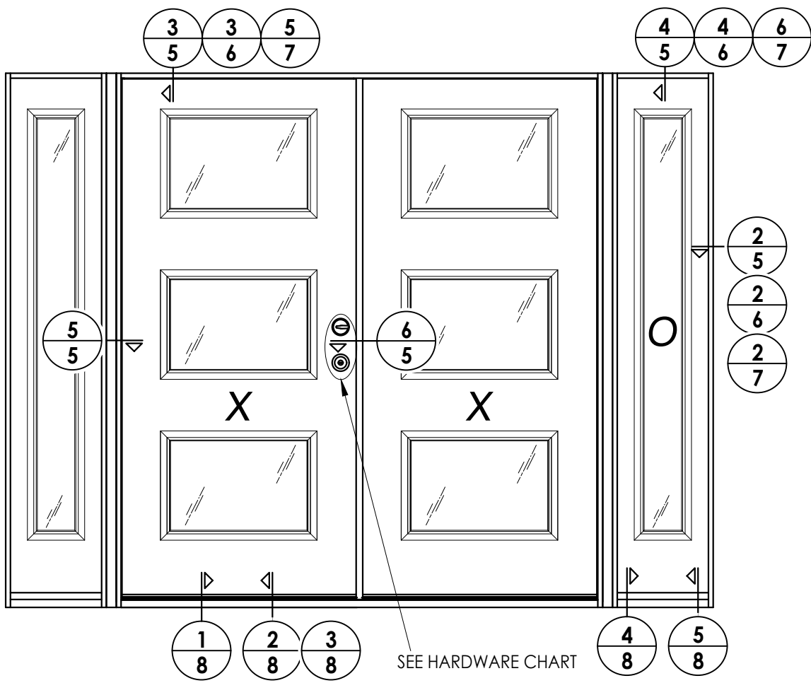
ELEVATION OX XO
